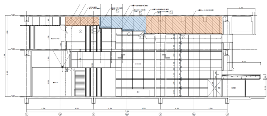
断面図
