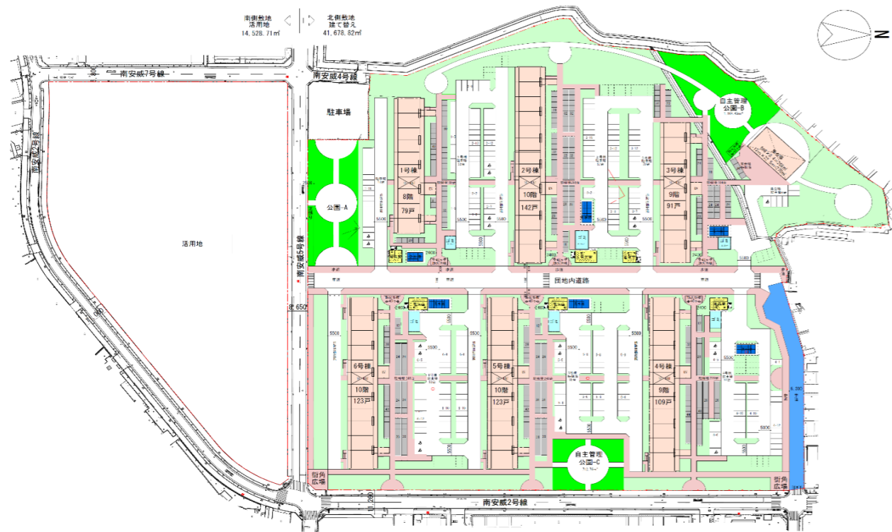
配置計画図
