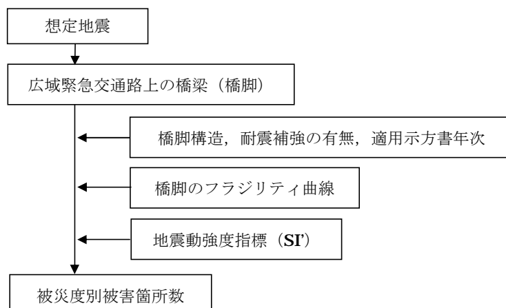
図 4-1 道路施設の被害想定フロー
